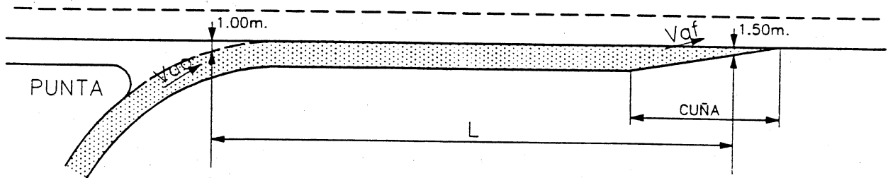
Figura 7.2 Carriles de cambio de velocidad.
