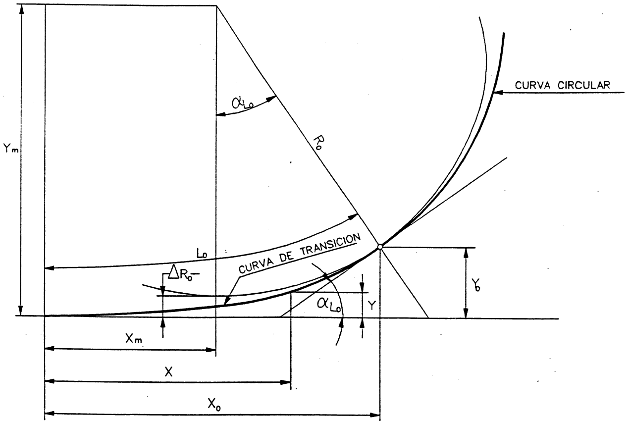
Figura 4.1 Curva de transición.
