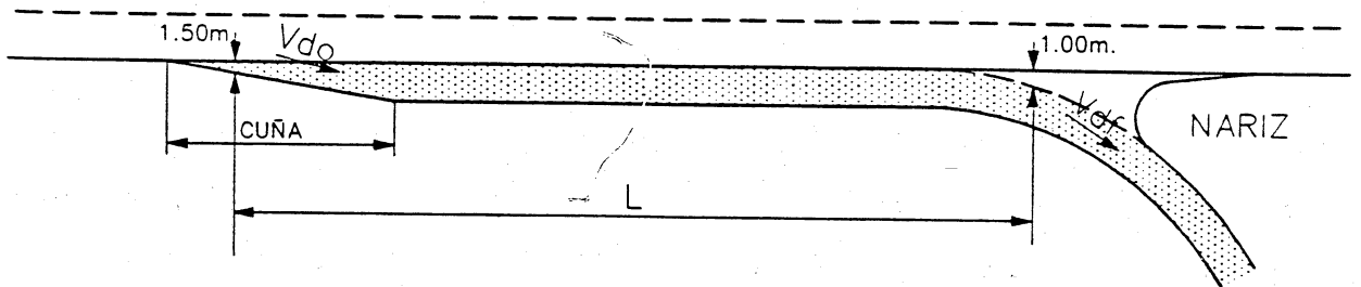
DECELERACION – TIPO PARALELO
