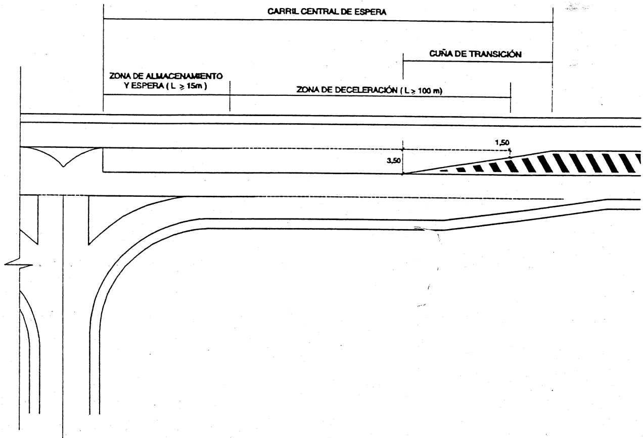
Figura 7.16 Carriles centrales de espera.
