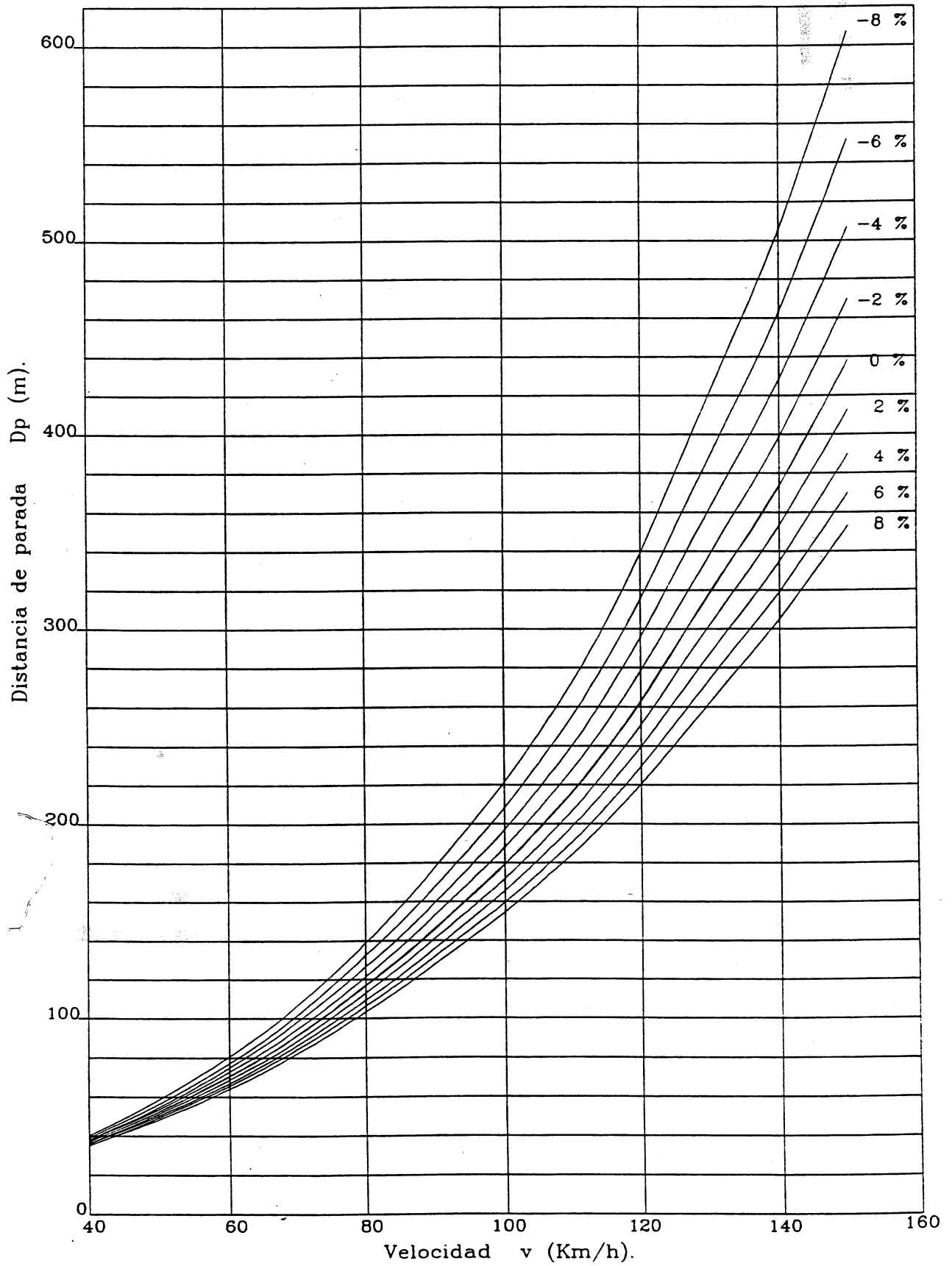
Figura 3.1 Distancia de parada.
