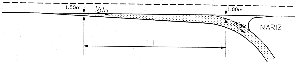
DECELERACION – TIPO DIRECTO
