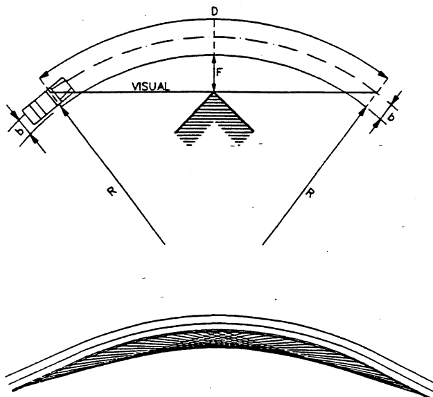
Figura 4.5 Visibilidad en curvas circulares.
