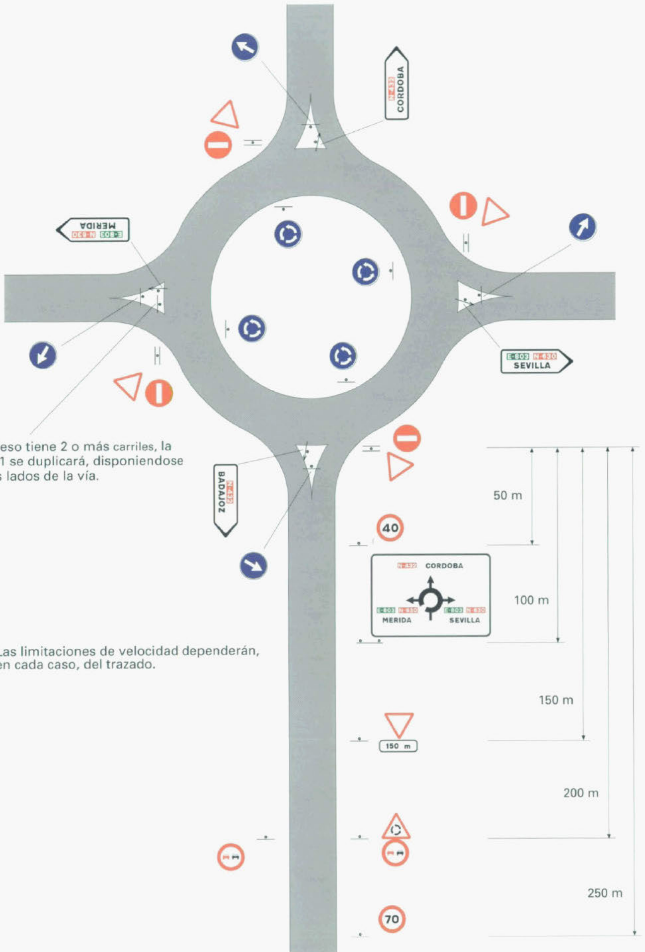
INTERSECCION EN GLORIETA
