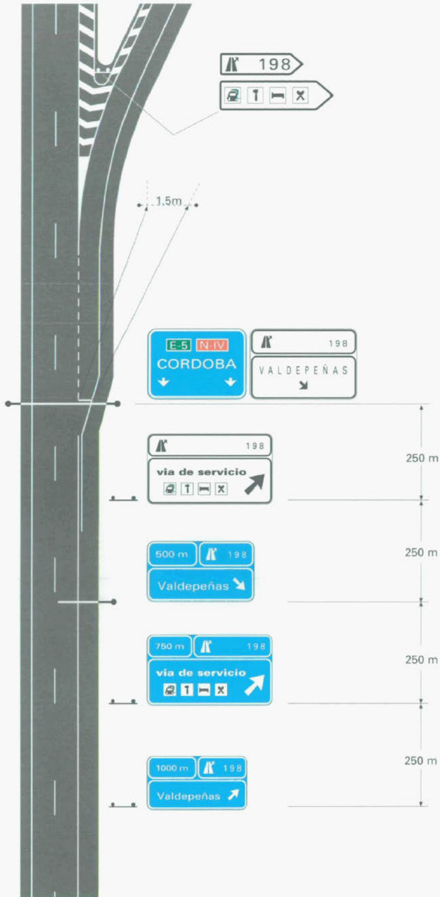
VIA DE SERVICIO CON SALIDA COMPARTIDA
