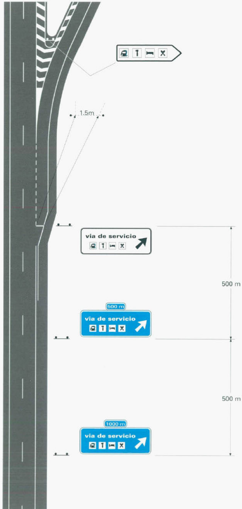
VIA DE SERVICIO CON SALIDA EXCLUSIVA
