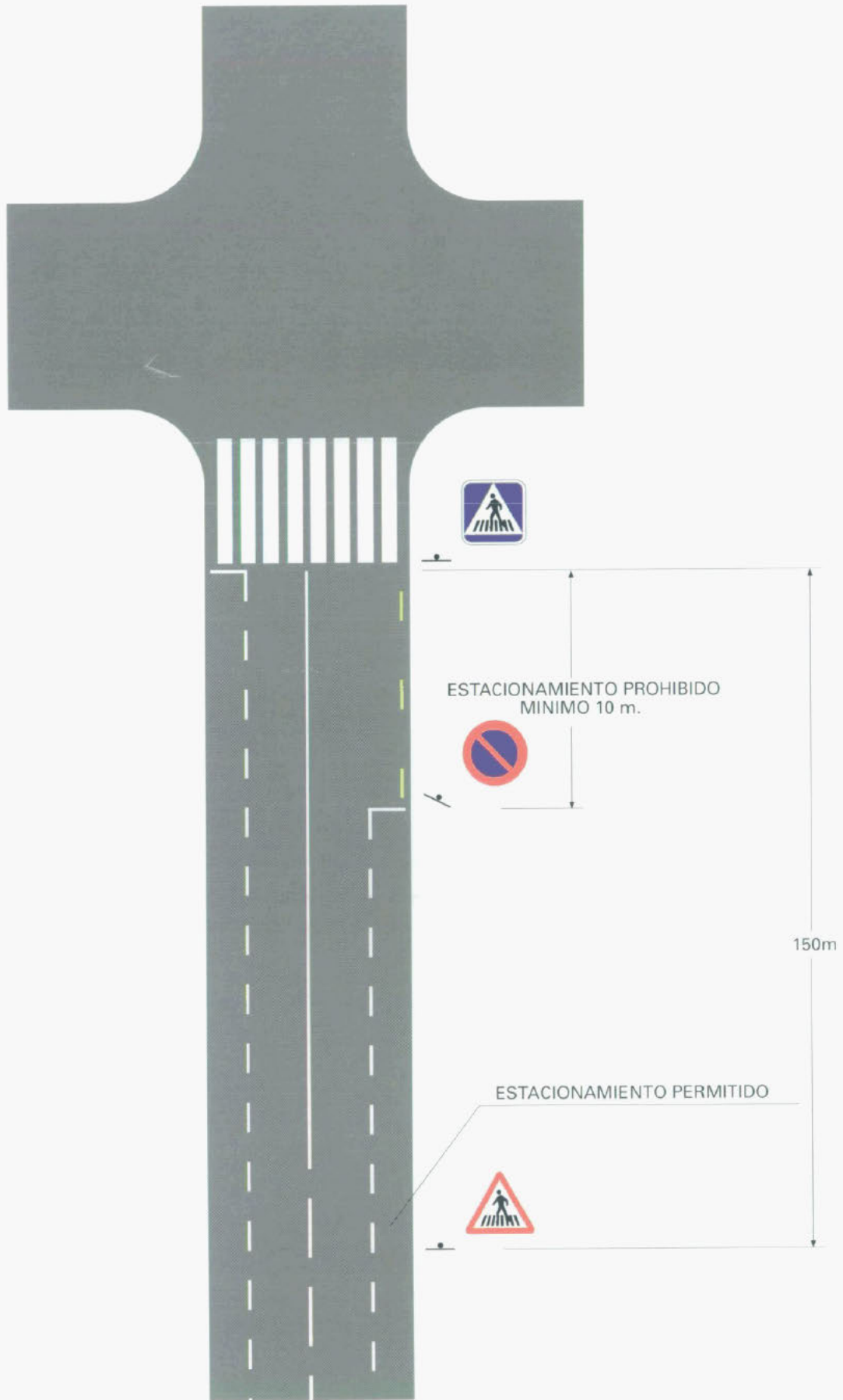
PASO DE PEATONES
