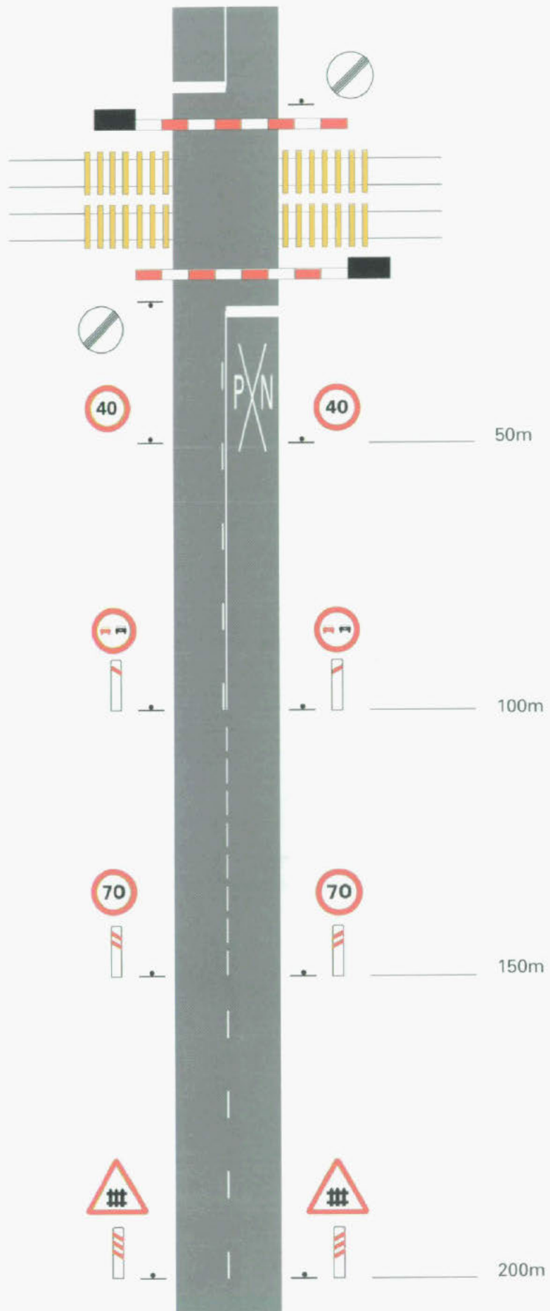
SEÑALIZACIÓN DE PASO A NIVEL CON BARRERA
