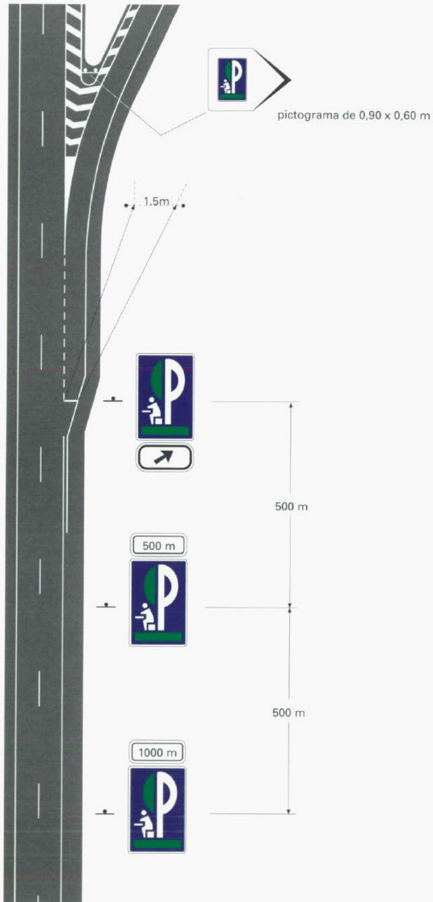
AREAS DE DESCANSO
