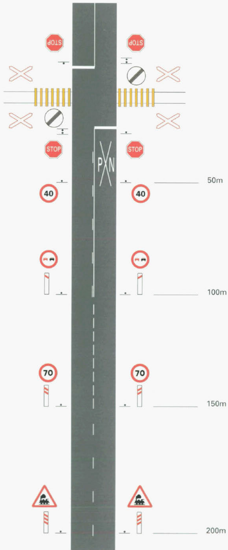
SEÑALIZACION DE PASO A NIVEL SIN BARRERA
