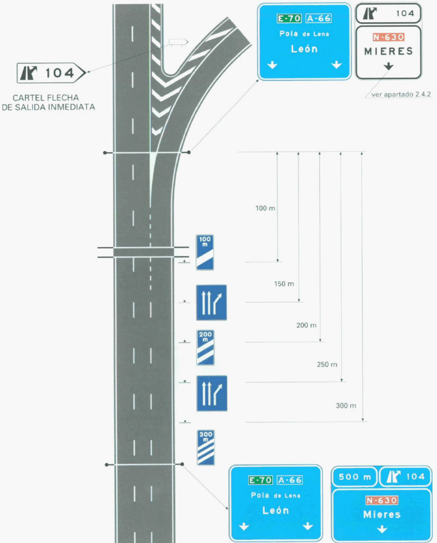
SALIDA CON PERDIDA DE CARRIL EN EL TRONCO
