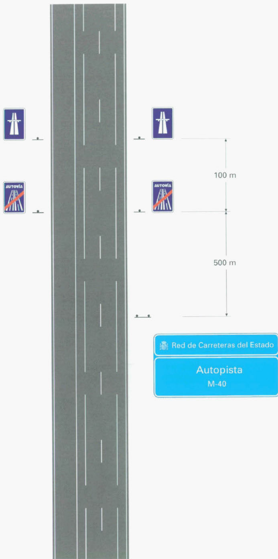
AUTOVIA - AUTOPISTA (CONEXION DIRECTA)
