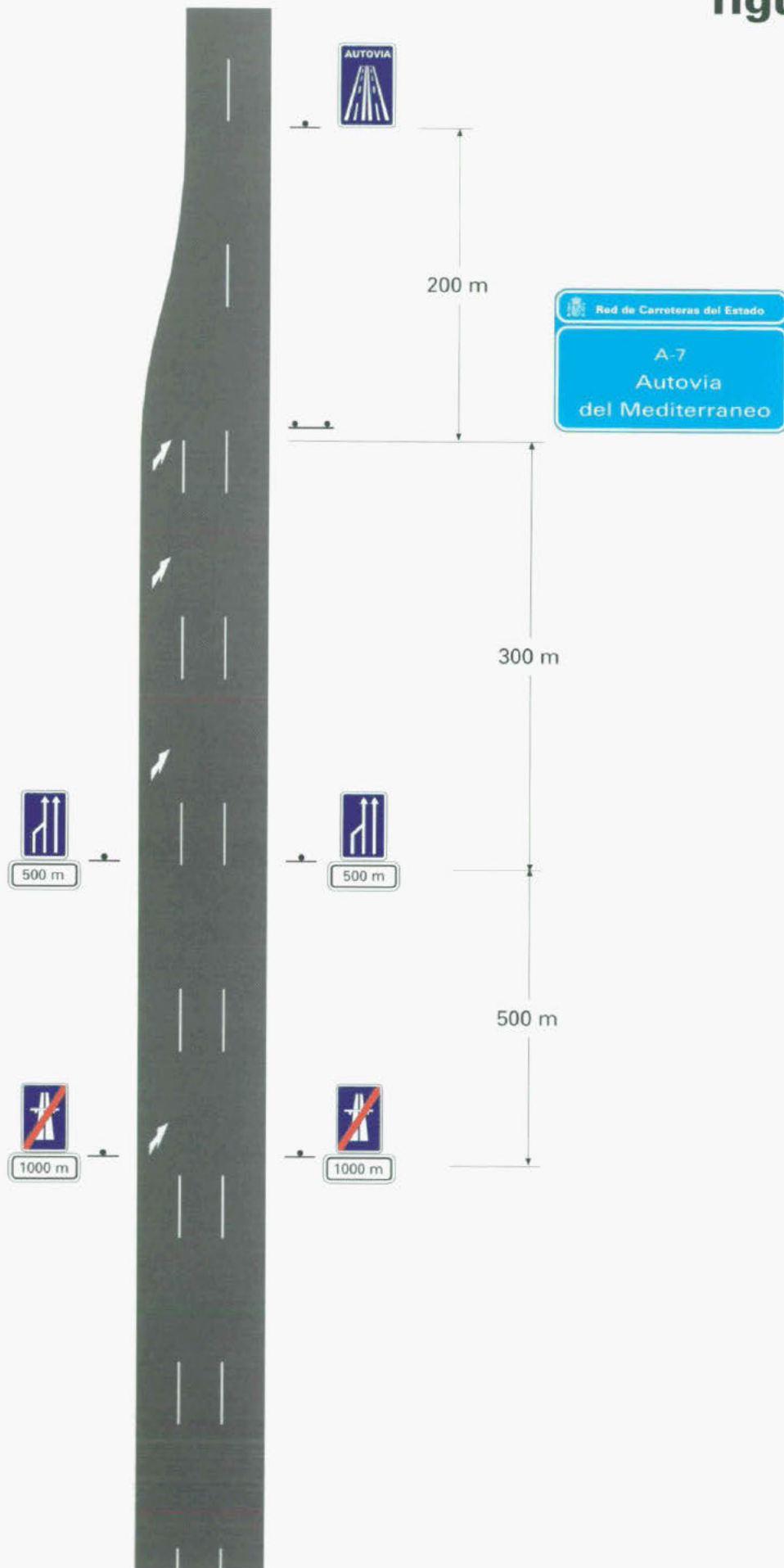
AUTOPISTA - AUTOVIA (CONEXION DIRECTA)
