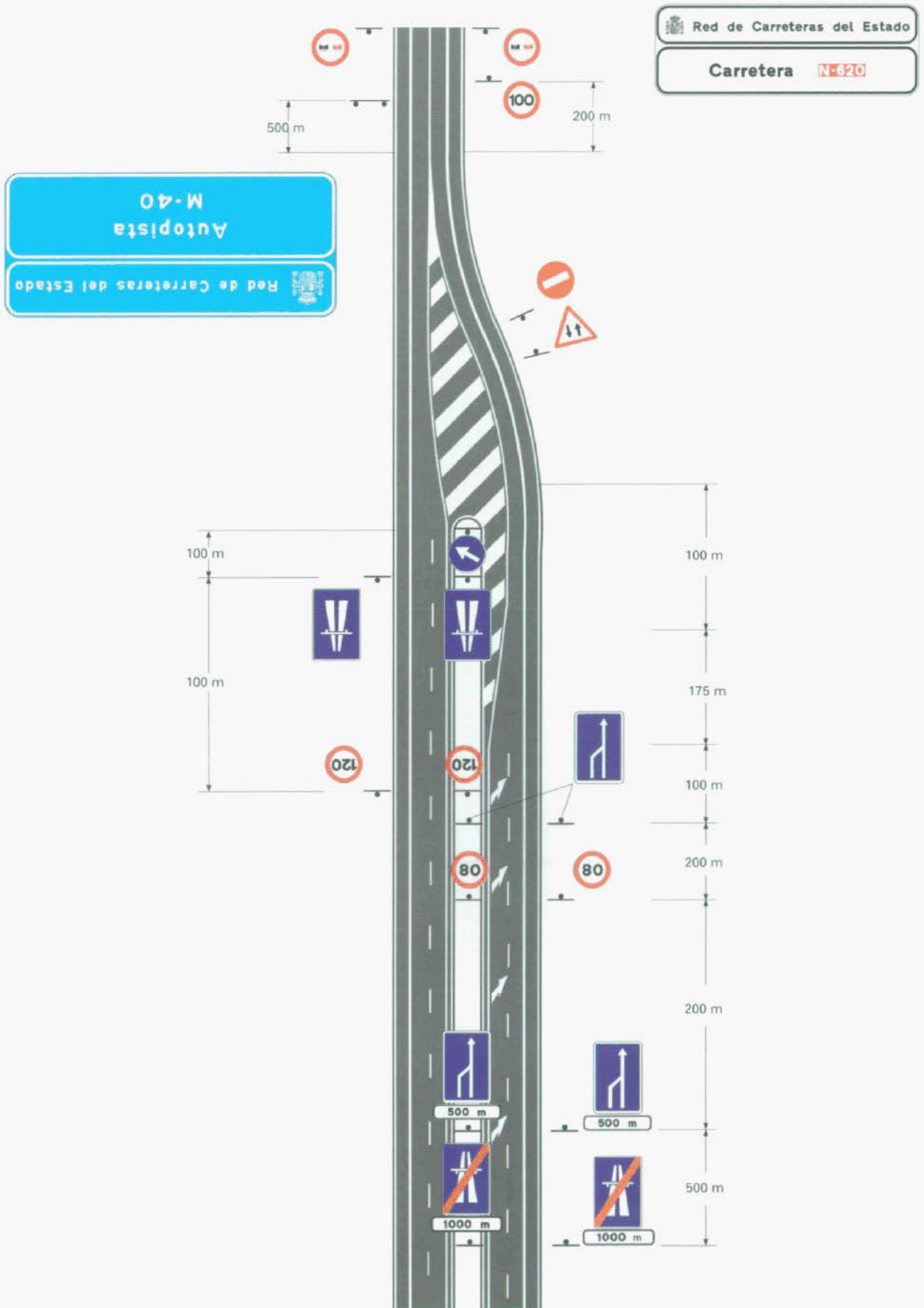
CONEXION DE AUTOPISTA CON CARRETERA CONVENCIONAL
