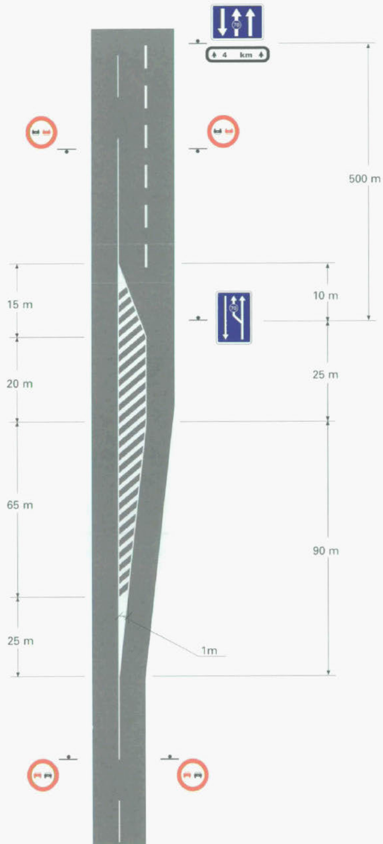
INICIO DE CARRIL ADICIONAL EN CARRETERA DE CALZADA UNICA
