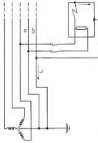
Figura 3. Esquema TN-S.
