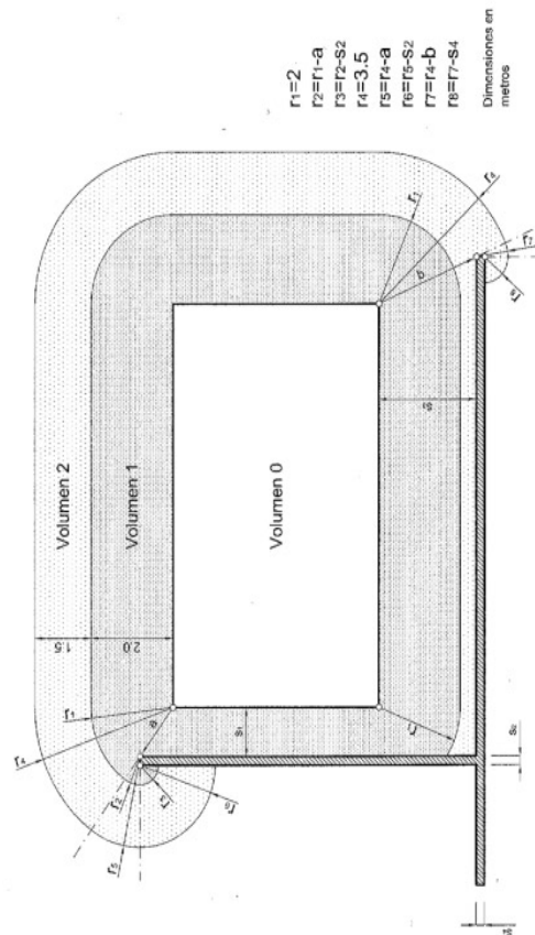
Figura 4. Volúmenes de protección en piscinas con paredes
