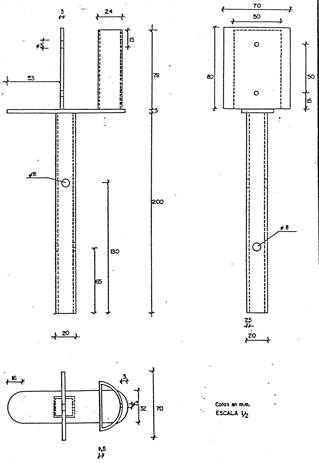
PE HITO DE ARISTA MODELO TIPO I PARA TERRENO DURO
